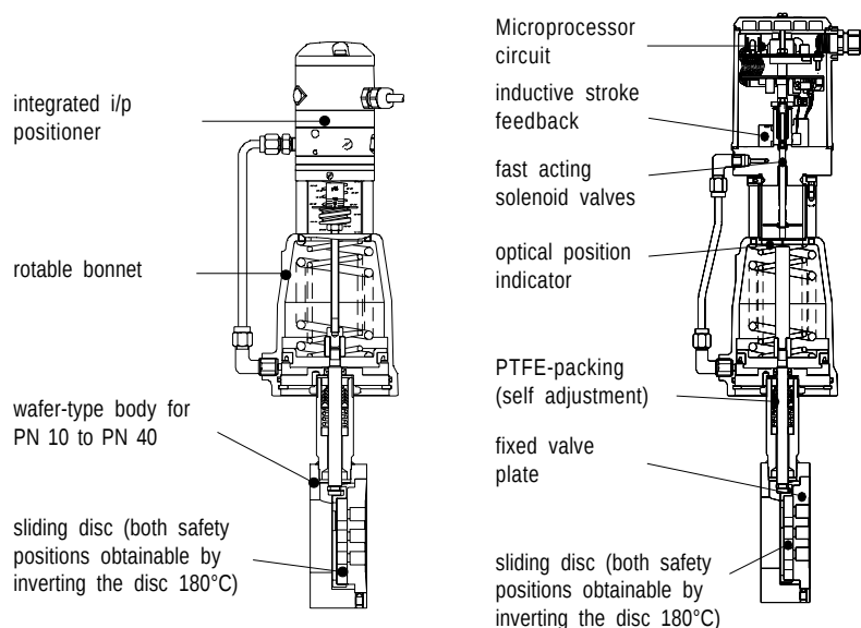
Type 8044 with i/p-positioner Typ 8047
